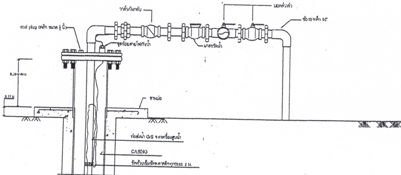
ภาพขยายการเดินท่อและสายไฟจากปากบ่อน้ำบาดาล
